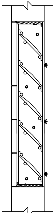
45° FIXED LOUVER BLADES
