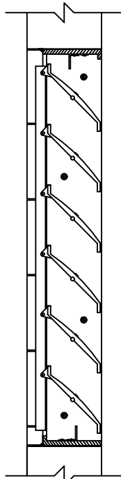
45° ADJUSTABLE LOUVER BLADES
